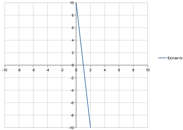
Wykres funkcji liniowej y=ax+b
